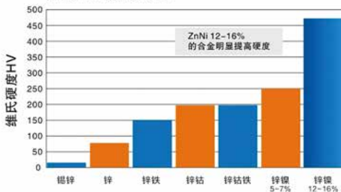
不同种类镀层的硬度
